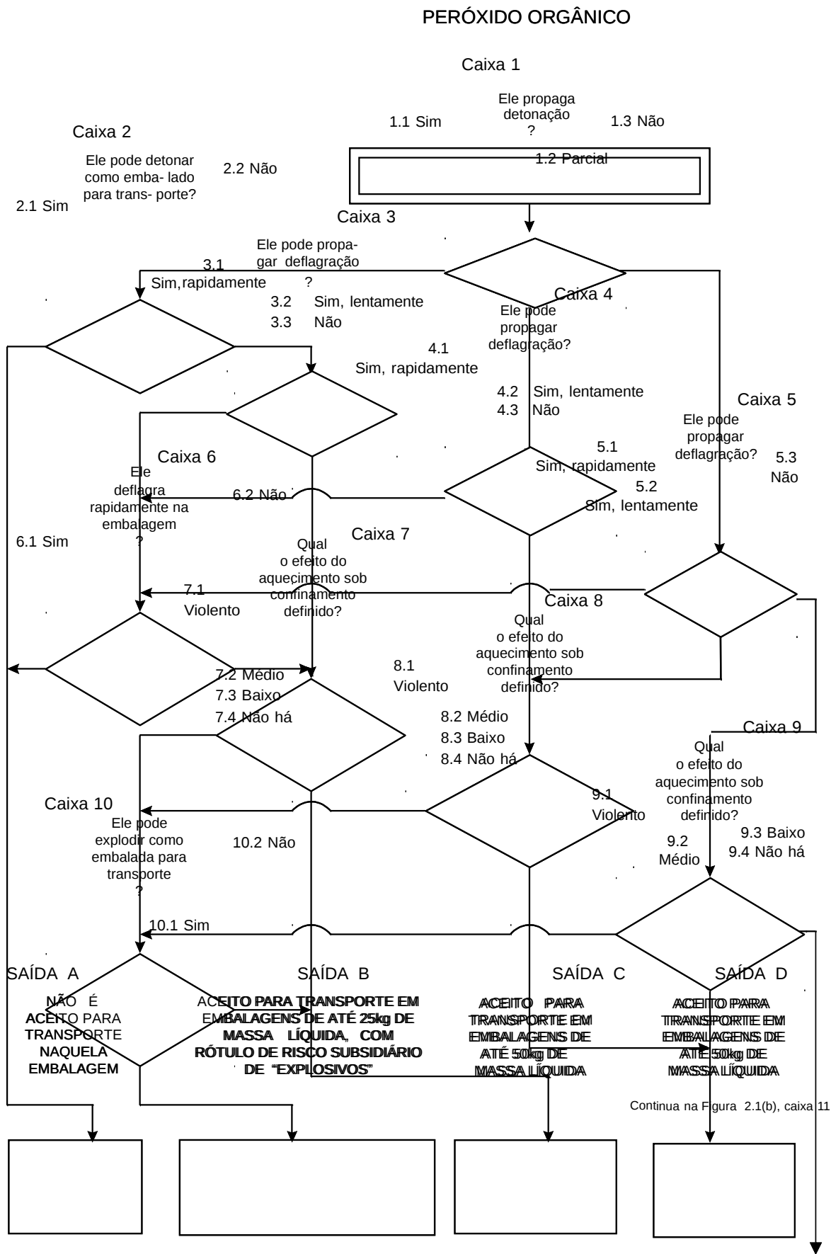
FIGURA 2.2 (a): FLUXOGRAMA PARA CLASSIFICAÇÃO DE PERÓXIDOS ORGÂNICOS
