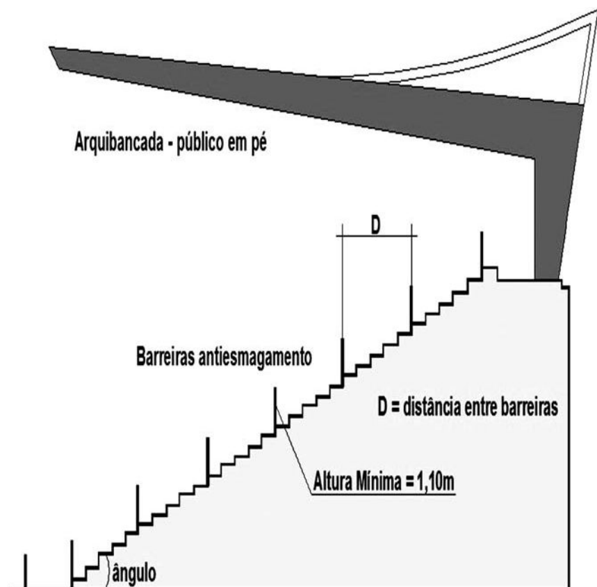
Resistência mecânica e distâncias entre barreiras antiesmagamentos
