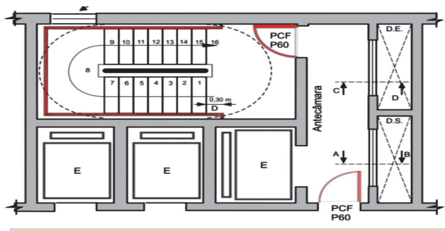
Figura 9: Escada enclausurada à prova de fumaça
