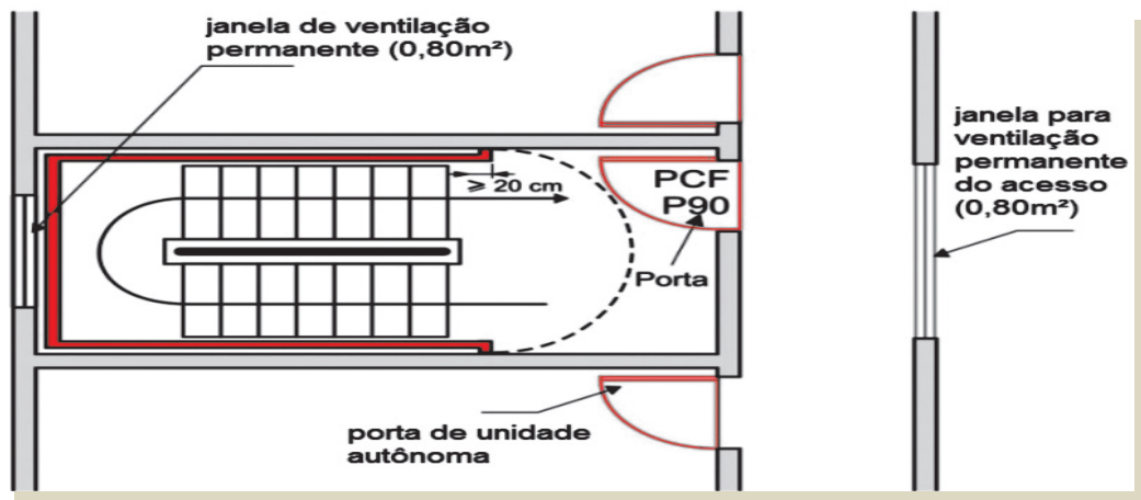
Figura 8: Ventilação da escada enclausurada protegida e seu acesso
