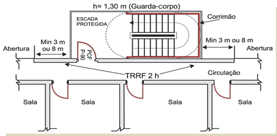
Figura 12: Escada aberta externa
