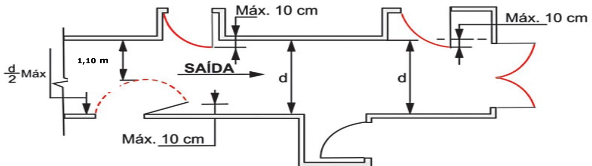
Figura 2: Abertura das portas no sentido de saída
