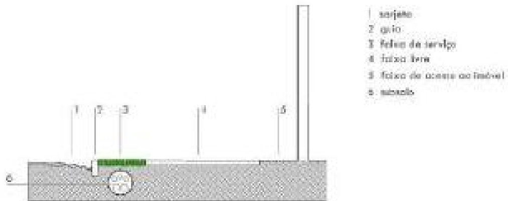
Figura 1. Faixas de composição da Calçada.
