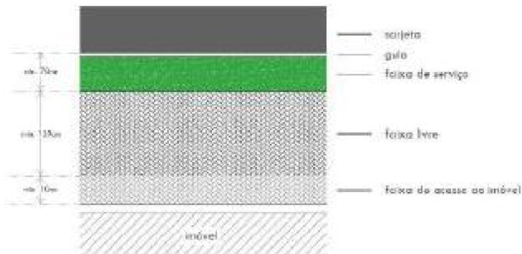
Figura 2. Elementos de composição da Calçada.
