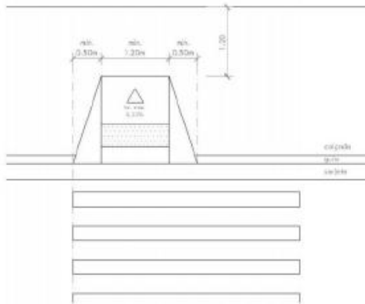
Figura 4. Dimensionamento mínimo para rampa de acessibilidade.
