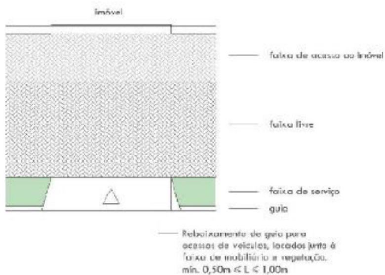
Figura 9. Rampas de acesso ao lote destinadas a veículos.
