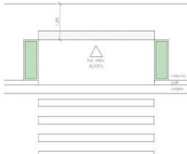
Figura 5. Rebordamento com extensão de faixa de travessia.
