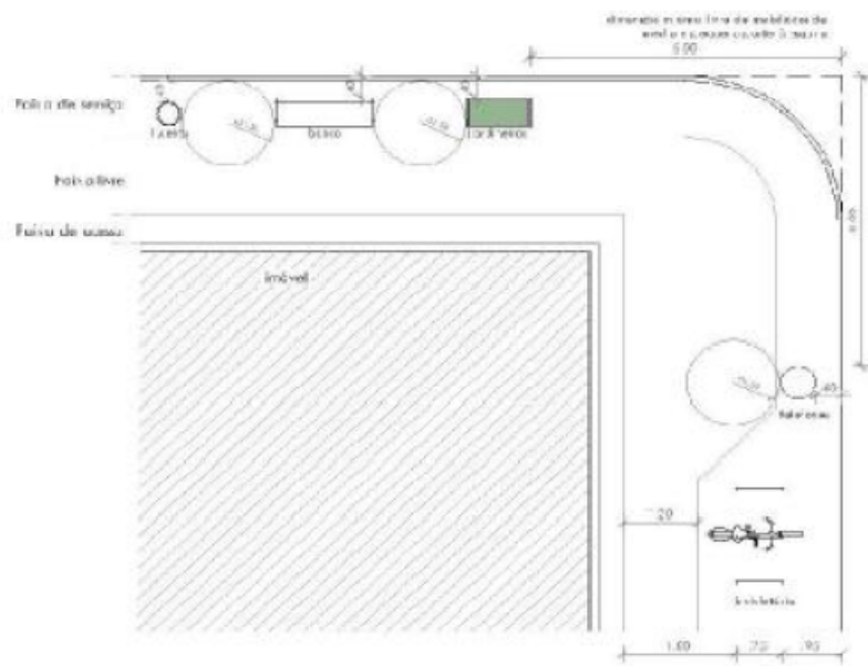
Figura 11. Localização de mobiliário de pequeno e médio porte (bancas, bancas, jardineiras, telefones públicos, bicicletários, etc.).
