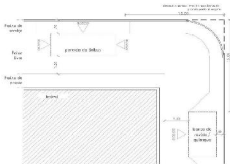
Figura 12. Localização de mobiliário de grande porte (parques de ônibus, bancas, quiosques, etc).
