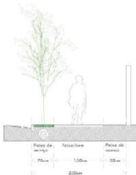
Figura 18. Dimensionamentos para faixas de Calçada do Padrão C em CORTE.
