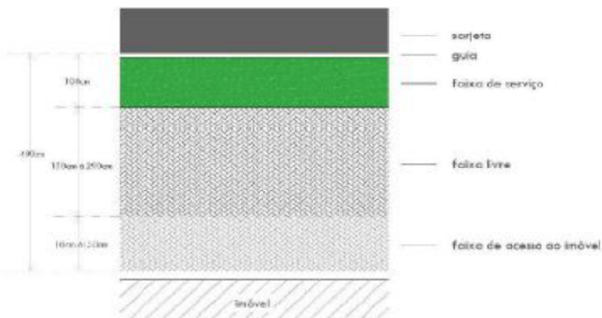
Figura 15. Dimensionamentos para faixas de Calçada do Padrão B.
