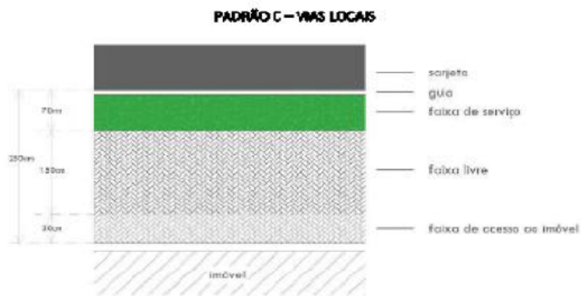
Figura 17. Dimensionamentos para faixas de Calçada do Padrão C.
