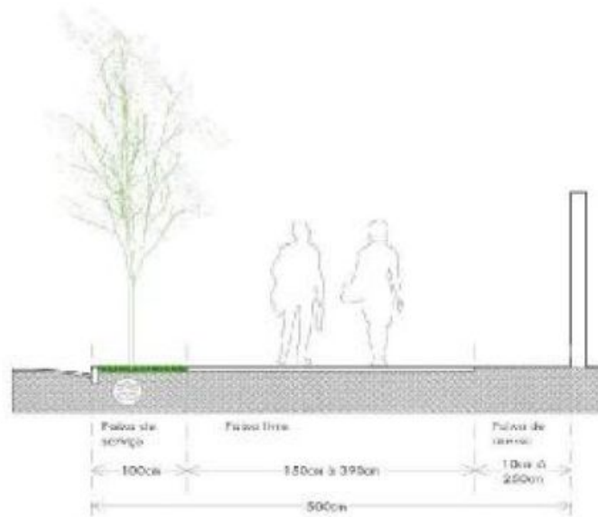
Figura 14. Dimensionamentos para faixas de Calçada do Padrão A em CORTE.
