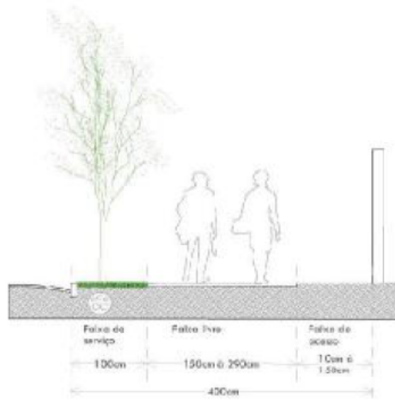
Figura 16. Dimensionamentos para faixas de Calçada do Padrão B em CORTE.
