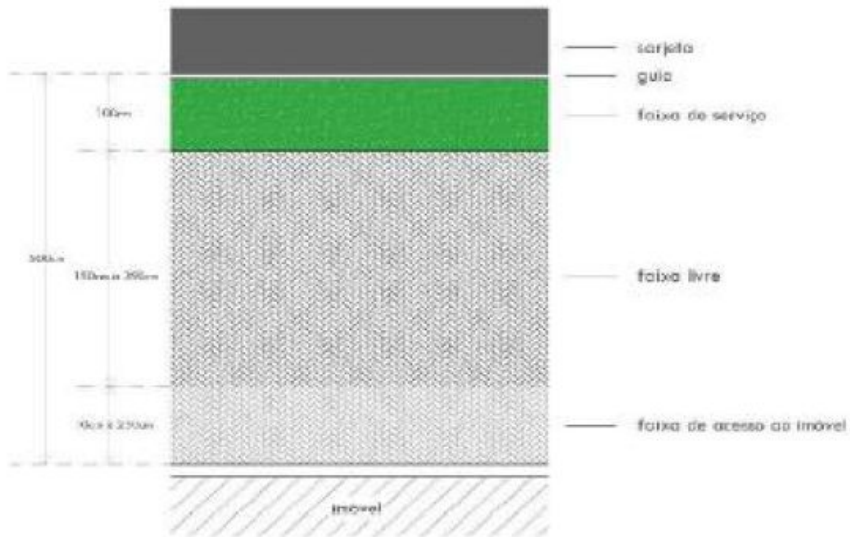
Figura 13. Dimensionamentos para faixas de calçada do Padrão A.
