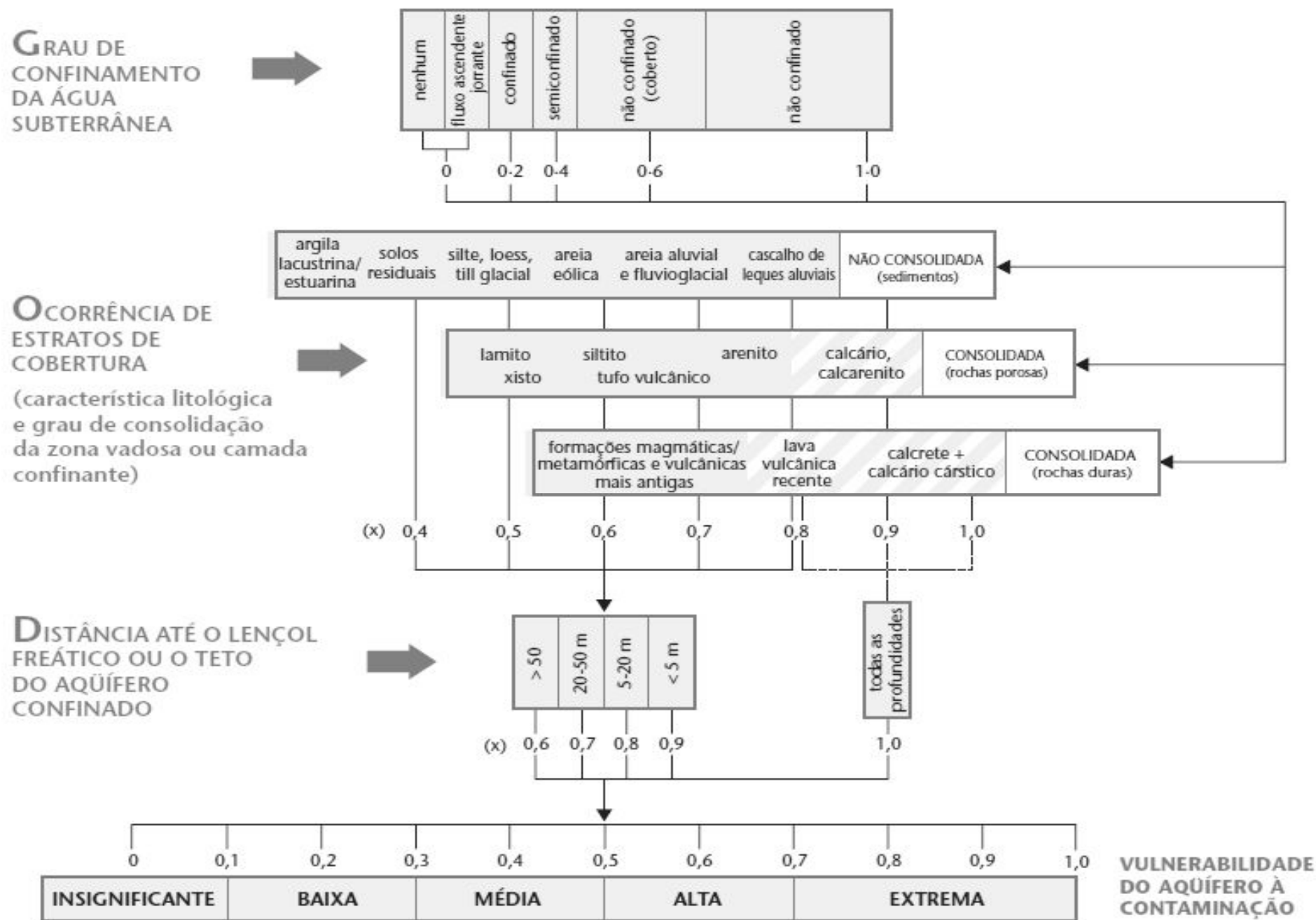
Figura 01 - Sistema GOD para avaliação da vulnerabilidade do aquífero à contaminação (Foster et al, 2006).
