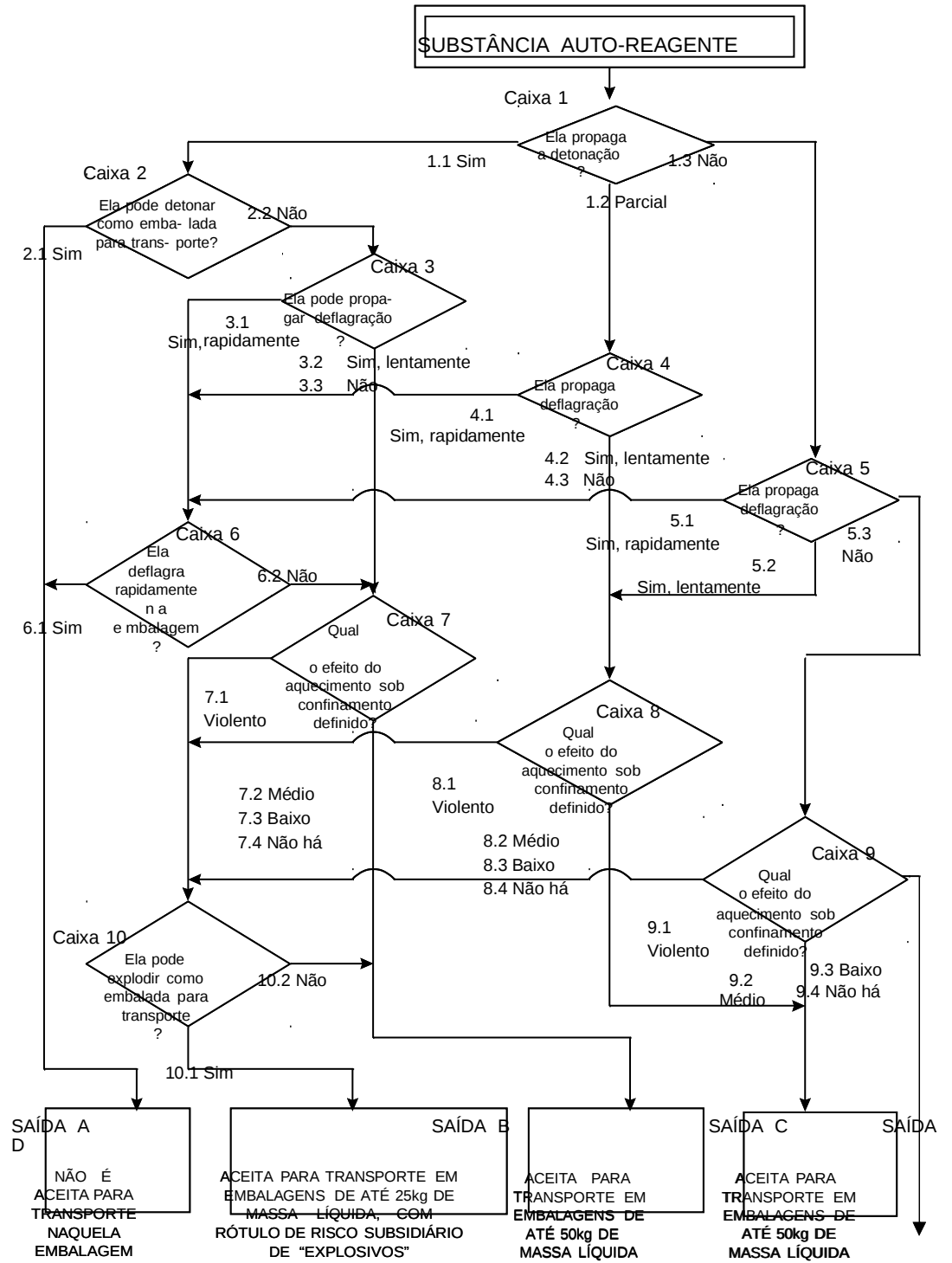
FIGURA 2.1 (a): FLUXOGRAMA PARA CLASSIFICAÇÃO DE SUBSTÂNCIAS AUTO-REAGENTES
