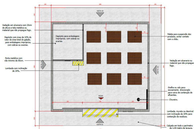
Imagem 5: Planta baixa do "modelo 2" do depósito de embalagens cheias de agrotóxicos na propriedade rural.
