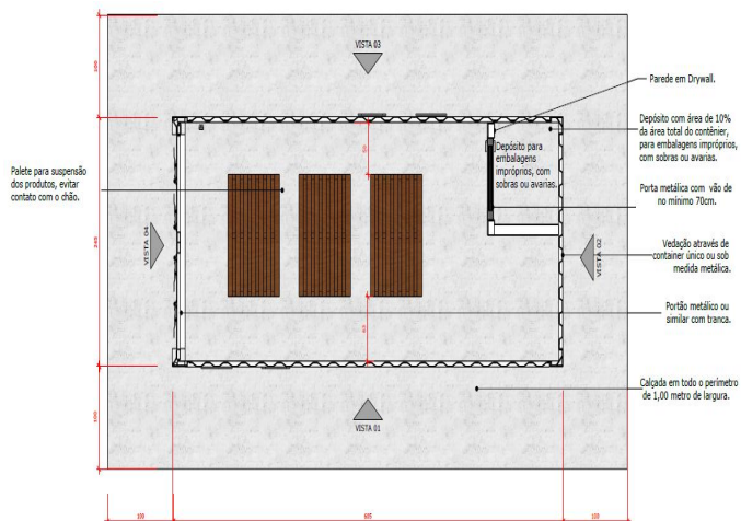
Imagem 10: Planta baixa do "modelo 3" (container) do depósito de embalagens cheias de agrotóxicos na propriedade rural.
