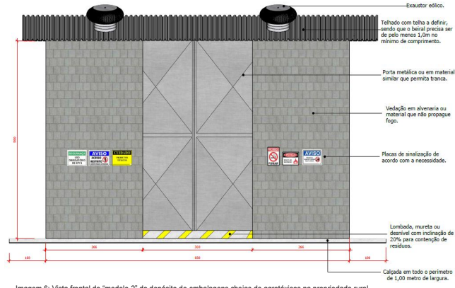
Imagem 6: Vista frontal do "modelo 2" do depósito de embalagens cheias de agrotóxicos na propriedade rural.
