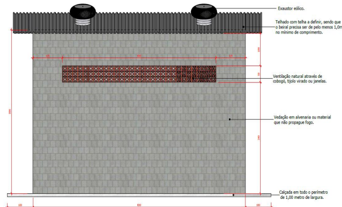
Imagem 8: Vista posterior do "modelo 2" do depósito de embalagens cheias de agrotóxicos na propriedade rural.
