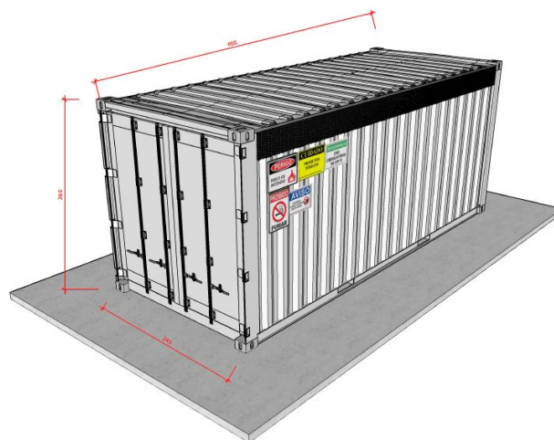
Imagem 9: Perspectiva do "modelo 3" (container) do depósito de embalagens cheias de agrotóxicos na propriedade rural.
