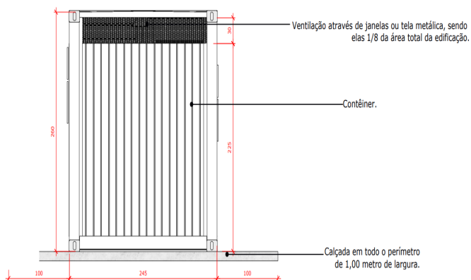
Imagem 13: Vista posterior do "modelo 3" (container) do depósito de embalagens cheias de agrotóxicos na propriedade rural.
