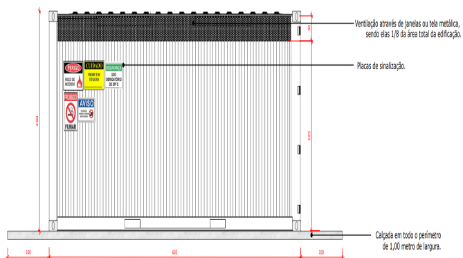
Imagem 12: Vista lateral do "modelo 3" (container) do depósito de embalagens cheias de agrotóxicos na propriedade rural.
