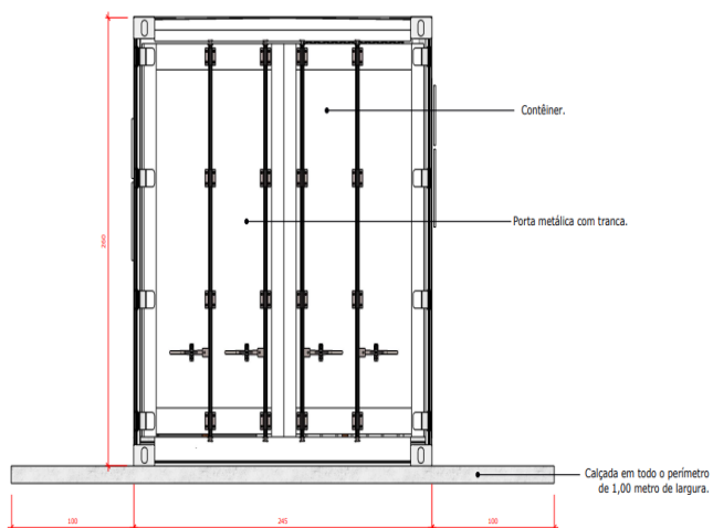
Imagem 11: Vista frontal do "modelo 3" (container) do depósito de embalagens cheias de agrotóxicos na propriedade rural.
