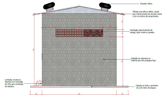
Imagem 7: Vista lateral do "modelo 2" do depósito de embalagens cheias de agrotóxicos na propriedade rural.
