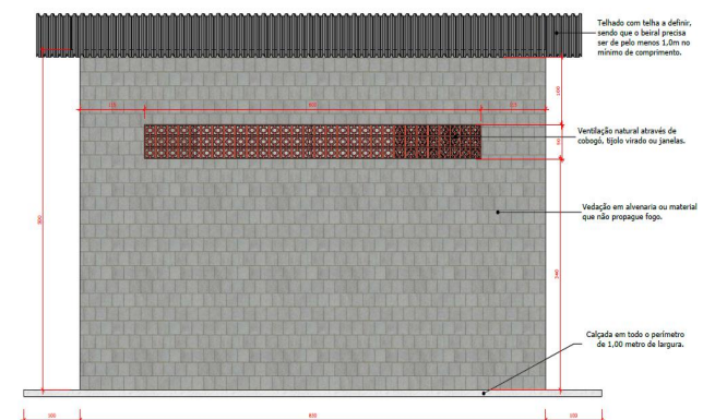
Imagem 4: Vista posterior do "modelo 1" do depósito de embalagens cheias de agrotóxicos na propriedade rural.
