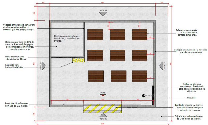
Imagem 1: Planta baixa do "modelo 1" do depósito de embalagens cheias de agrotóxicos na propriedade rural.
