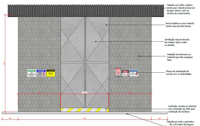
Imagem 2: Vista frontal do "modelo 1" do depósito de embalagens cheias de agrotóxicos na propriedade rural.
