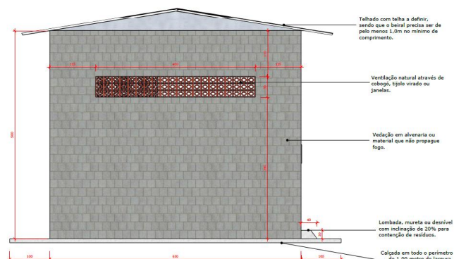
Imagem 3: Vista lateral "modelo 1" do depósito de embalagens cheias de agrotóxicos na propriedade rural.
