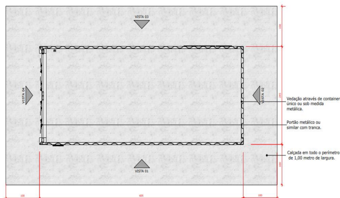
Imagem 23: Planta baixa do "modelo 3" (container) do depósito de embalagens vazias de agrotóxicos na propriedade rural.
