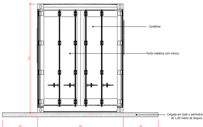
Imagem 24: Vista frontal do "modelo 3" (container) do depósito de embalagens vazias de agrotóxicos na propriedade rural.
