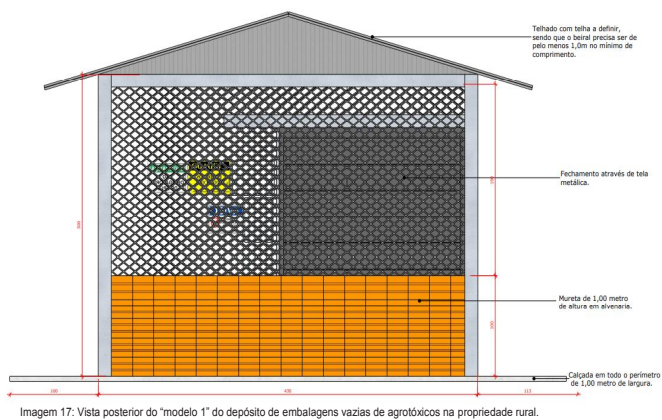
Imagem 17: Vista posterior do "modelo 1" do depósito de embalagens vazias de agrotóxicos na propriedade rural.
