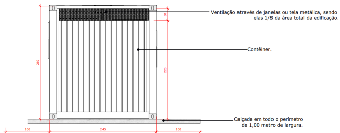
Imagem 26: Vista posterior do "modelo 3" (container) do depósito de embalagens vazias de agrotóxicos na propriedade rural.
