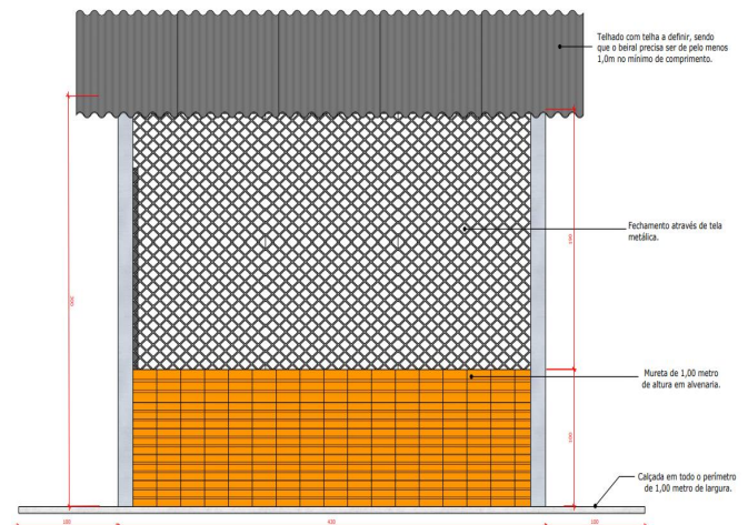
Imagem 15: Vista frontal do "modelo 1" do depósito de embalagens vazias de agrotóxicos na propriedade rural.
