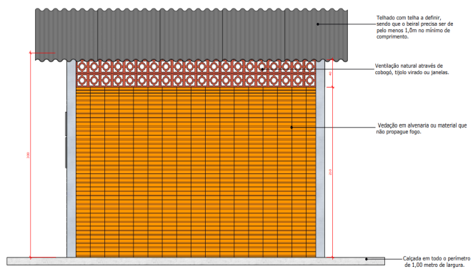
Imagem 20: Vista lateral do "modelo 2" do depósito de embalagens vazias de agrotóxicos na propriedade rural.
