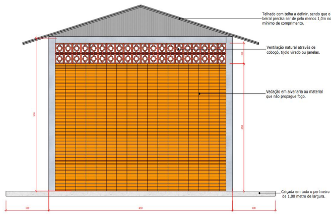
Imagem 21: Vista posterior do "modelo 2" do depósito de embalagens vazias de agrotóxicos na propriedade rural.
