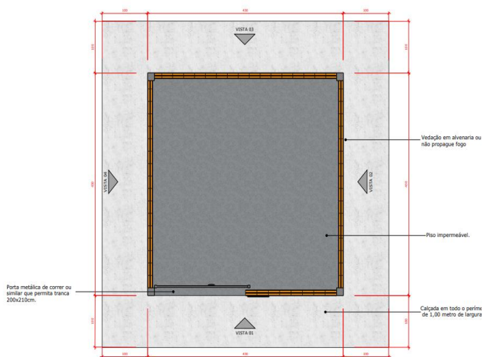
Imagem 18: Planta baixa do "modelo 2" do depósito de embalagens vazias de agrotóxicos na propriedade rural.
