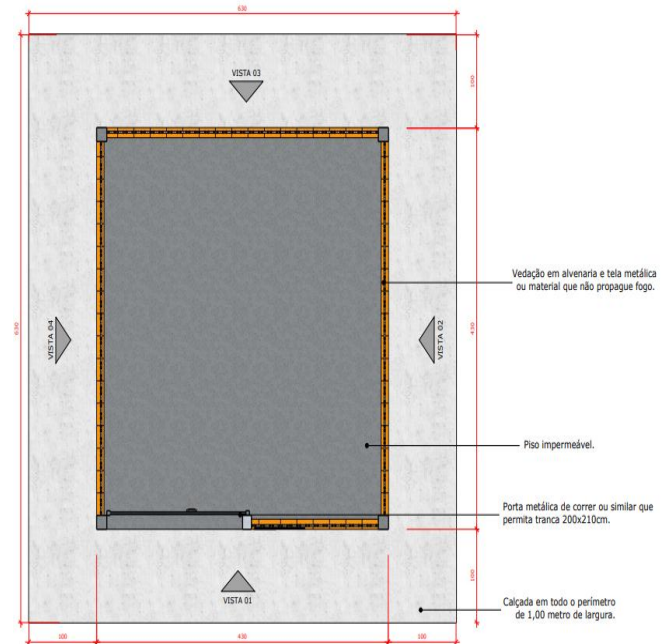
Imagem 14: Planta baixa do "modelo 1" do depósito de embalagens vazias de agrotóxicos na propriedade rural.
