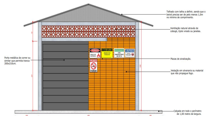
Imagem 19: Vista frontal do "modelo 2" do depósito de embalagens vazias de agrotóxicos na propriedade rural.
