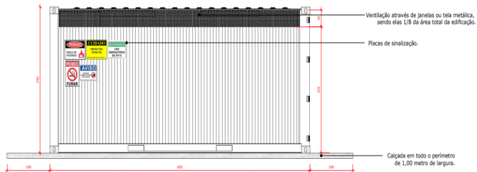
Imagem 25: Vista lateral do "modelo 3" (container) do depósito de embalagens vazias de agrotóxicos na propriedade rural.
