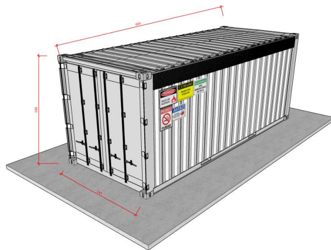
Imagem 22: Imagem em perspectiva do "modelo 3" (container) do depósito de embalagens vazias de agrotóxicos na propriedade rural.
