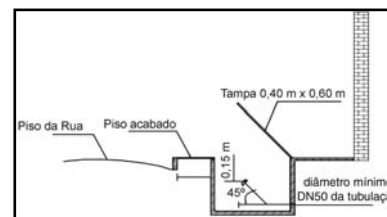
Figura 2: Dispositivo de recalque no passeio público
