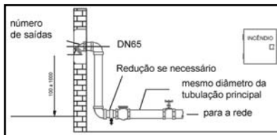
Figura 1: Dispositivo de recalque tipo coluna
