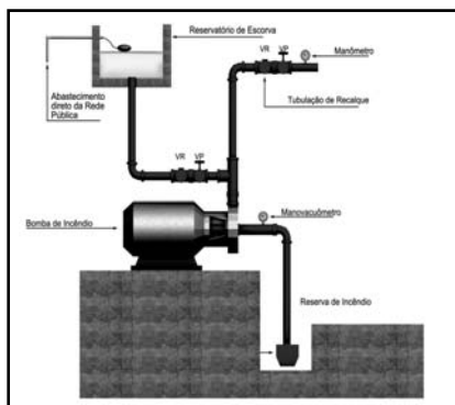
Figura C.3: Exemplo de afogamento de bomba de incêndio
