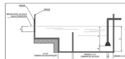
Figura B.5 – Alimentação natural do reservatório por canal
