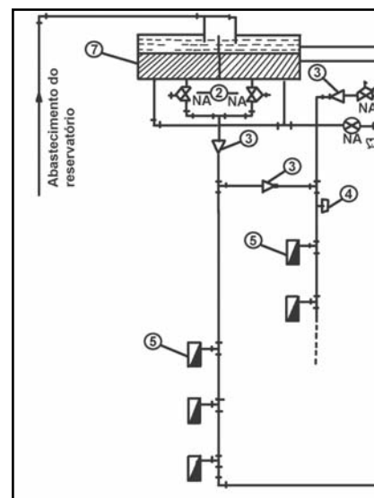
Figura C.6: Esquema de instalação de bomba de reforço abastecendo os pontos de hidrantes ou mangotinhos mais desfavoráveis considerados no cálculo, (prumada específica)
