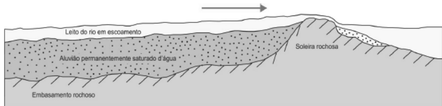
FIGURA 1 – Corte longitudinal de um rio onde uma ondulação do embasamento rochoso proporcionou o acúmulo de aluviões a montante, saturado durante o ano. A seta evidencia o sentido de escoamento do rio.
