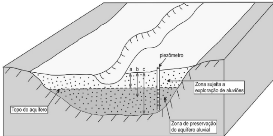
FIGURA 2 – Avaliação da zona de exploração de aluviões: (a) profundidade do nível hidrostático (topo do aquífero); (b) 50% da espessura do depósito aluvial; (c) espessura total do depósito aluvial.
