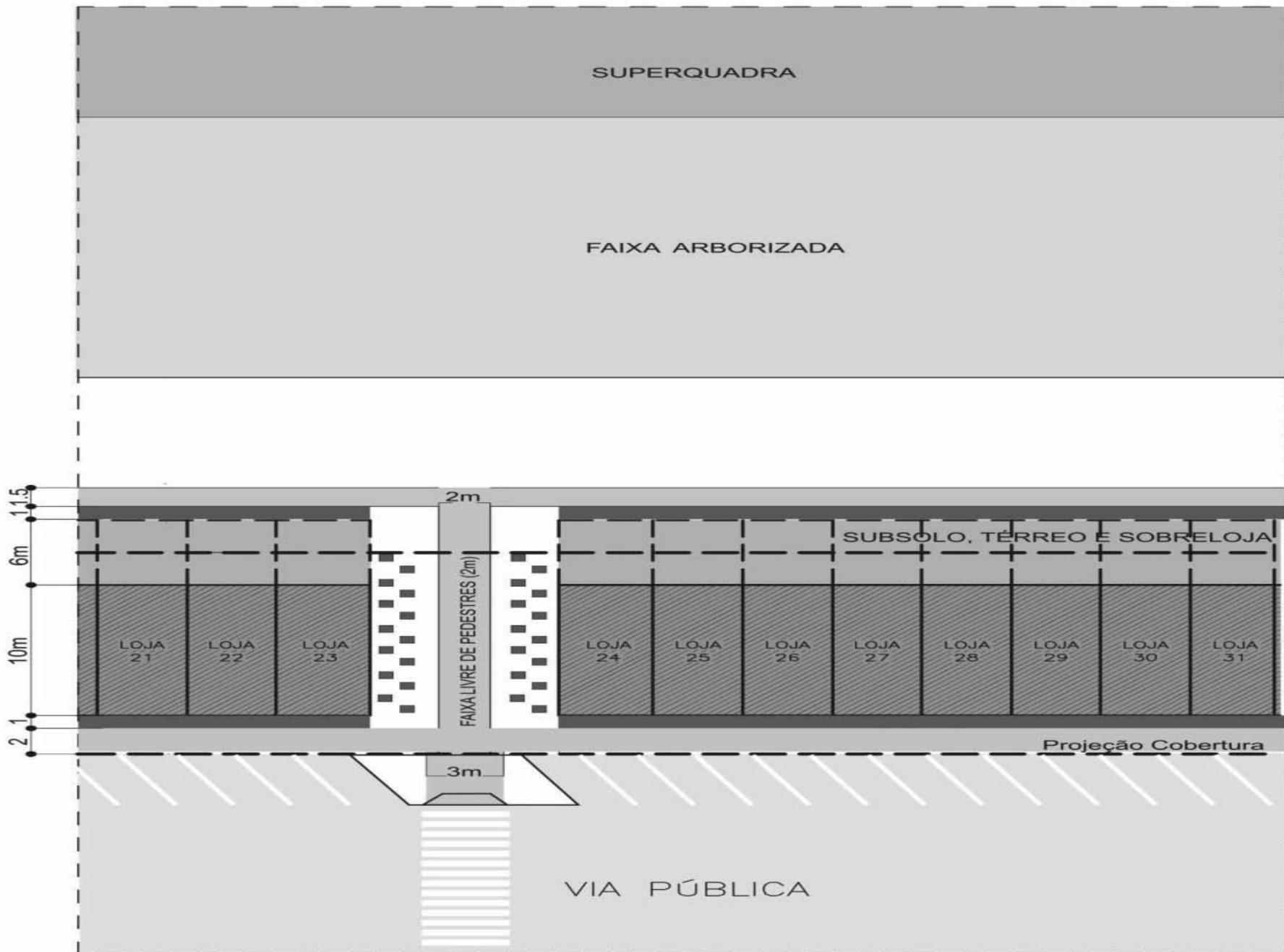
PLANTA - COMERCIAL LOCAL SUL SEM ESCALA
