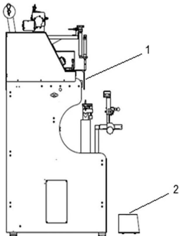
Legenda: 1. dispositivo de obstrução 2. proteção fixa do pedal de acionamento Figura 19: Máquina de montar base de calçados - vista lateral
