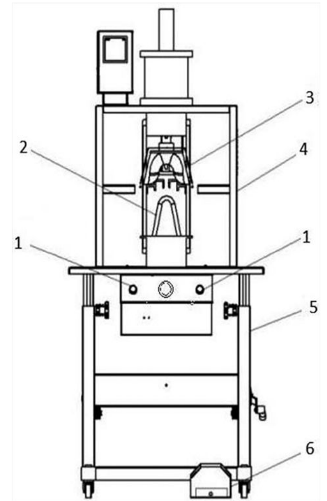
Figura 7: Máquina de cambrê com borrachão - Vista Frontal
