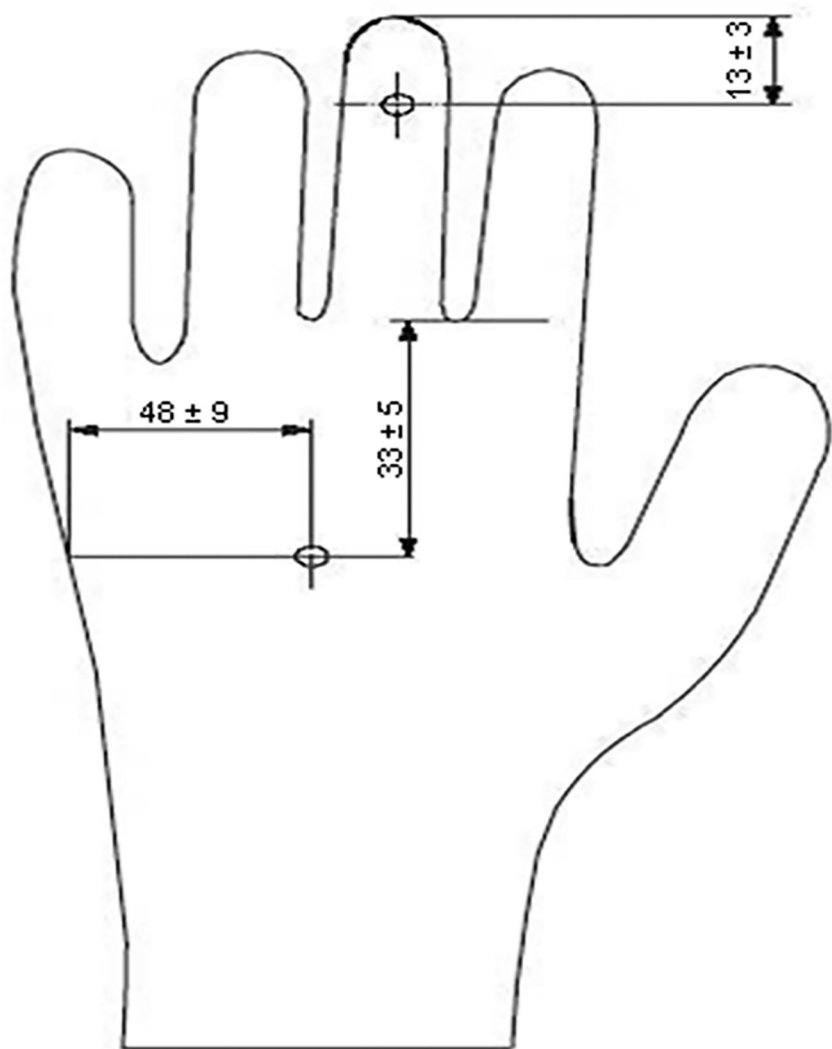
Figura A.2 - Pontos de medição para espessura da luva
