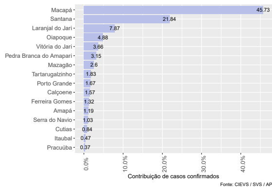
(a) Semana Epidemiológica - 14
