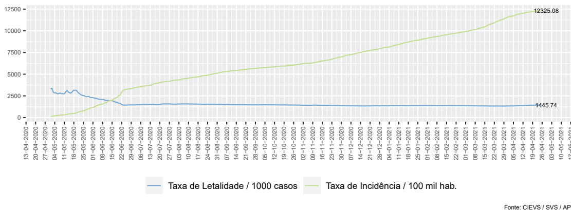
Figure 6: COVID-19: Evolução temporal da taxa de incidência versus letalidade no Estado do Amapá
