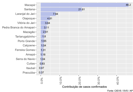
(b) Semana Epidemiológica - 15
