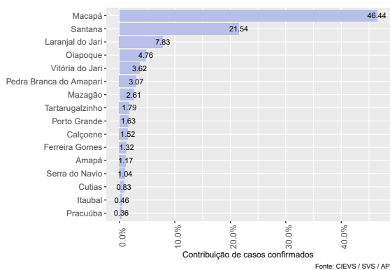
(c) Semana Epidemiológica - 16
