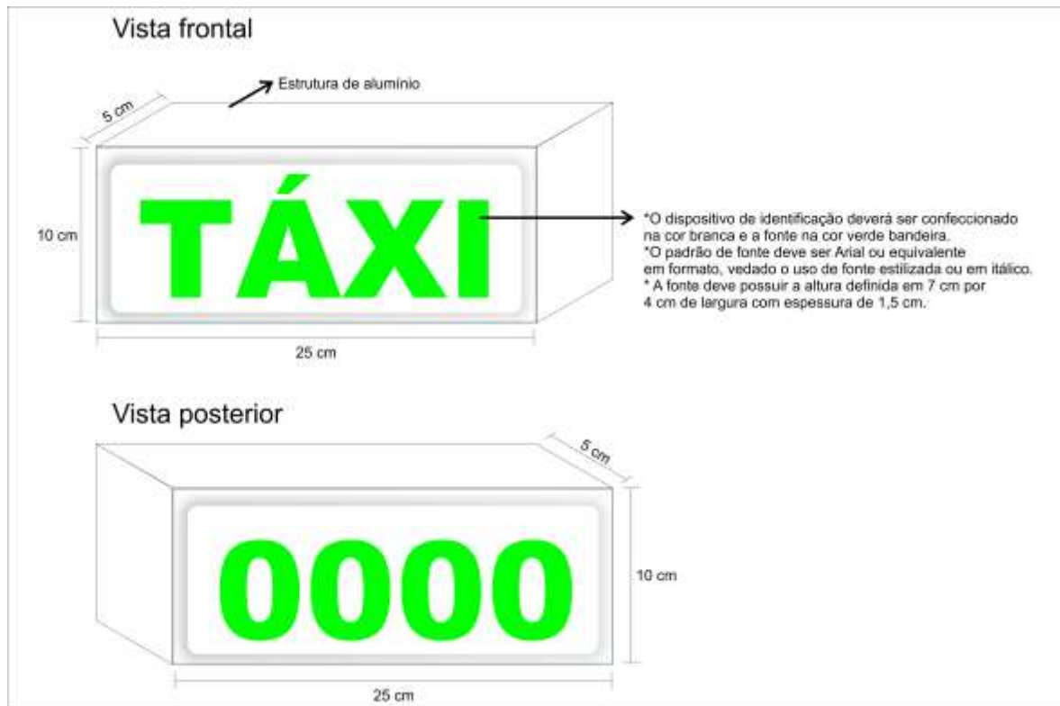
Figura 1: Luminoso Convencional (25cm)
