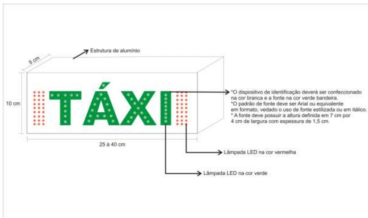
Figura 1: Esquema de lâmpadas – vista anterior
