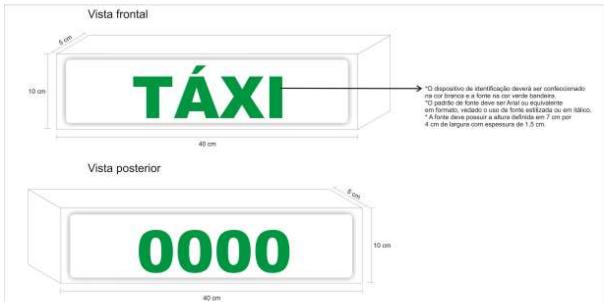
Figura 2: Luminoso Convencional (40cm)
