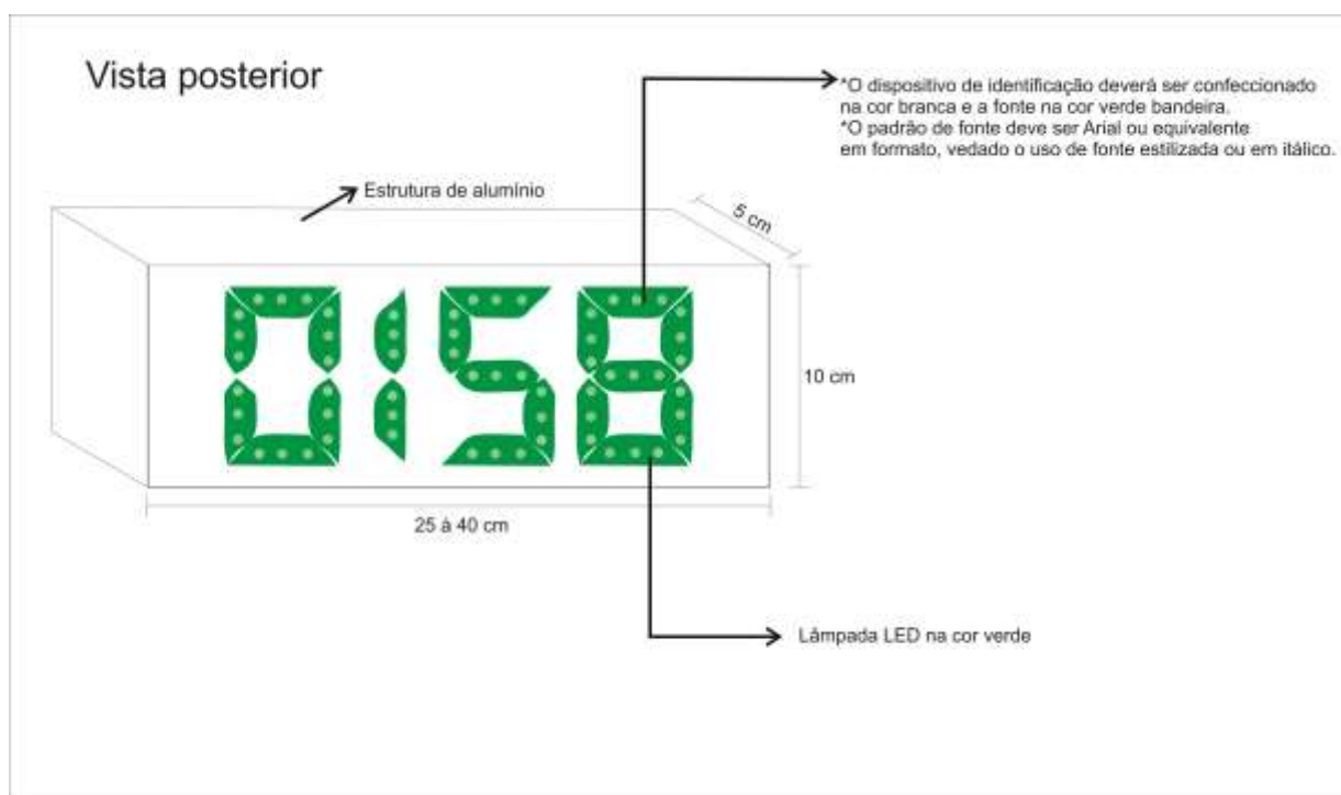
Figura 2: Esquema de lâmpadas – vista posterior
