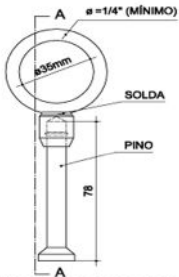
1 TRANSPASSADOR DE CABO - VISTA FRONTAL
