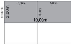
Figura 2- Dois Módulos - 3,00x10,00m, justaposição pelo lado menor – frente lado menor
