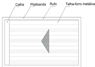
PLANTA COBERTURA QUIOSQUE tipologia 1
