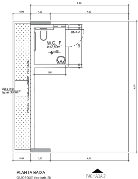
PLANTA BAIXA QUIOSQUE tipologia 2b
