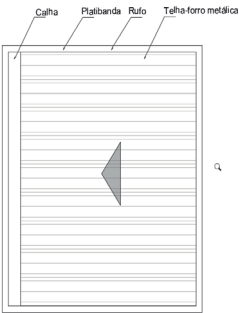
PLANTA COBERTURA QUIOSQUE tipologia 2b
