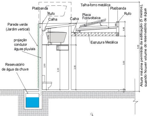
CORTE esquemático C.C. QUIOSQUE tipologia 2b
