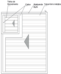
PLANTA COBERTURA com volume de água QUIOSQUE tipologia 2b
